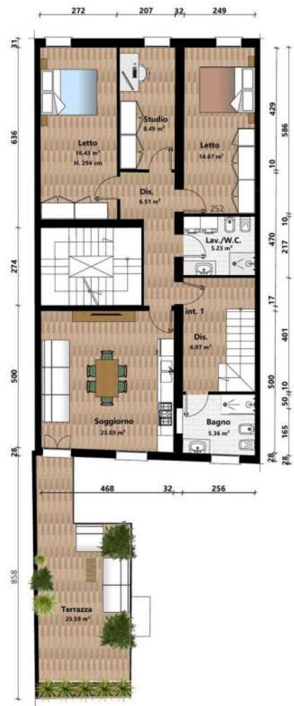
PIANO PRIMO Scala 1:100
