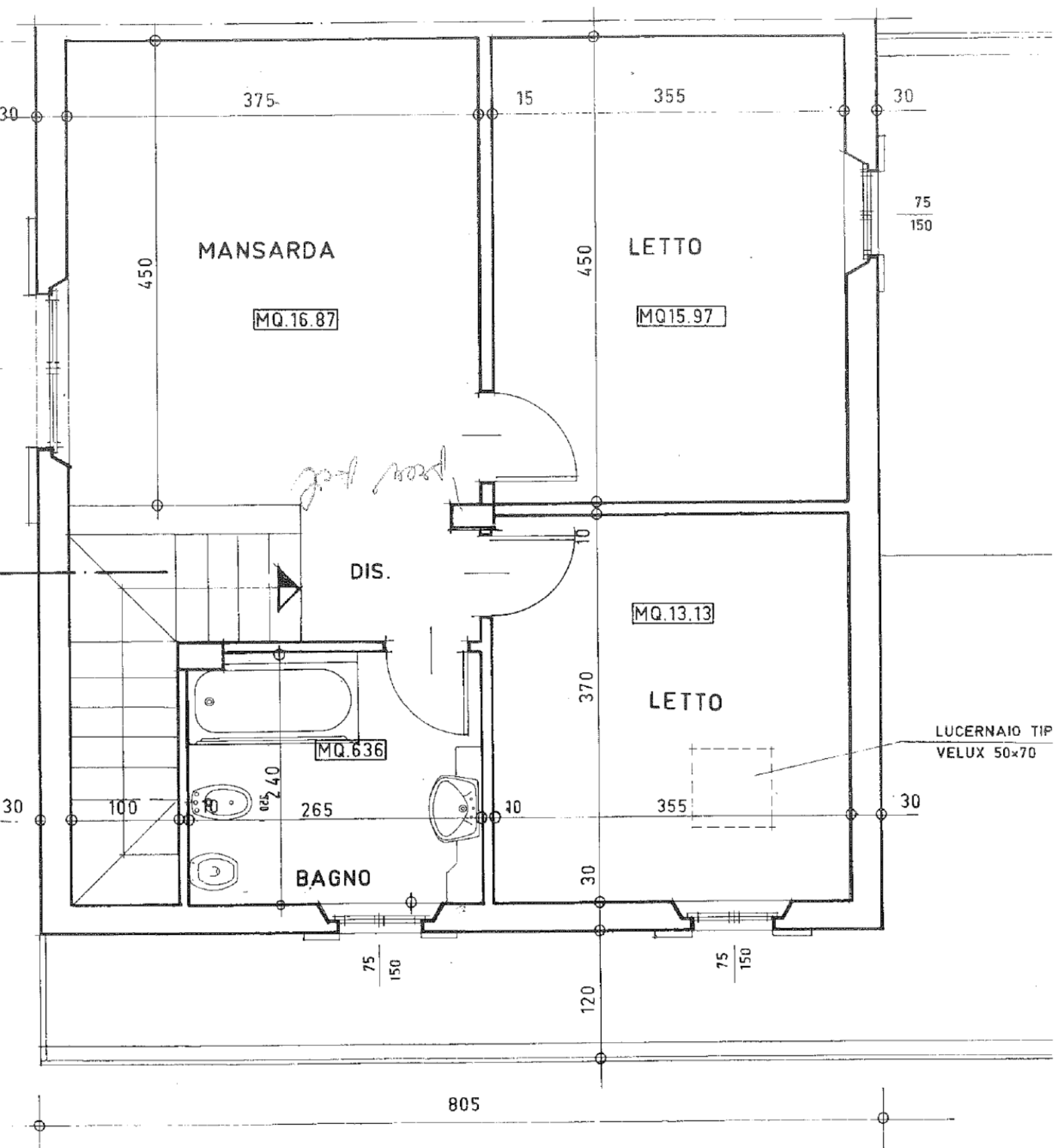
PIANO PRIMO
