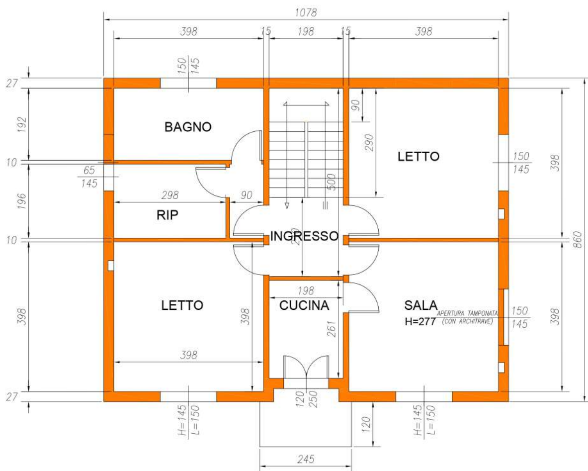
PIANO PRIMO (STATO ATTUALE)
