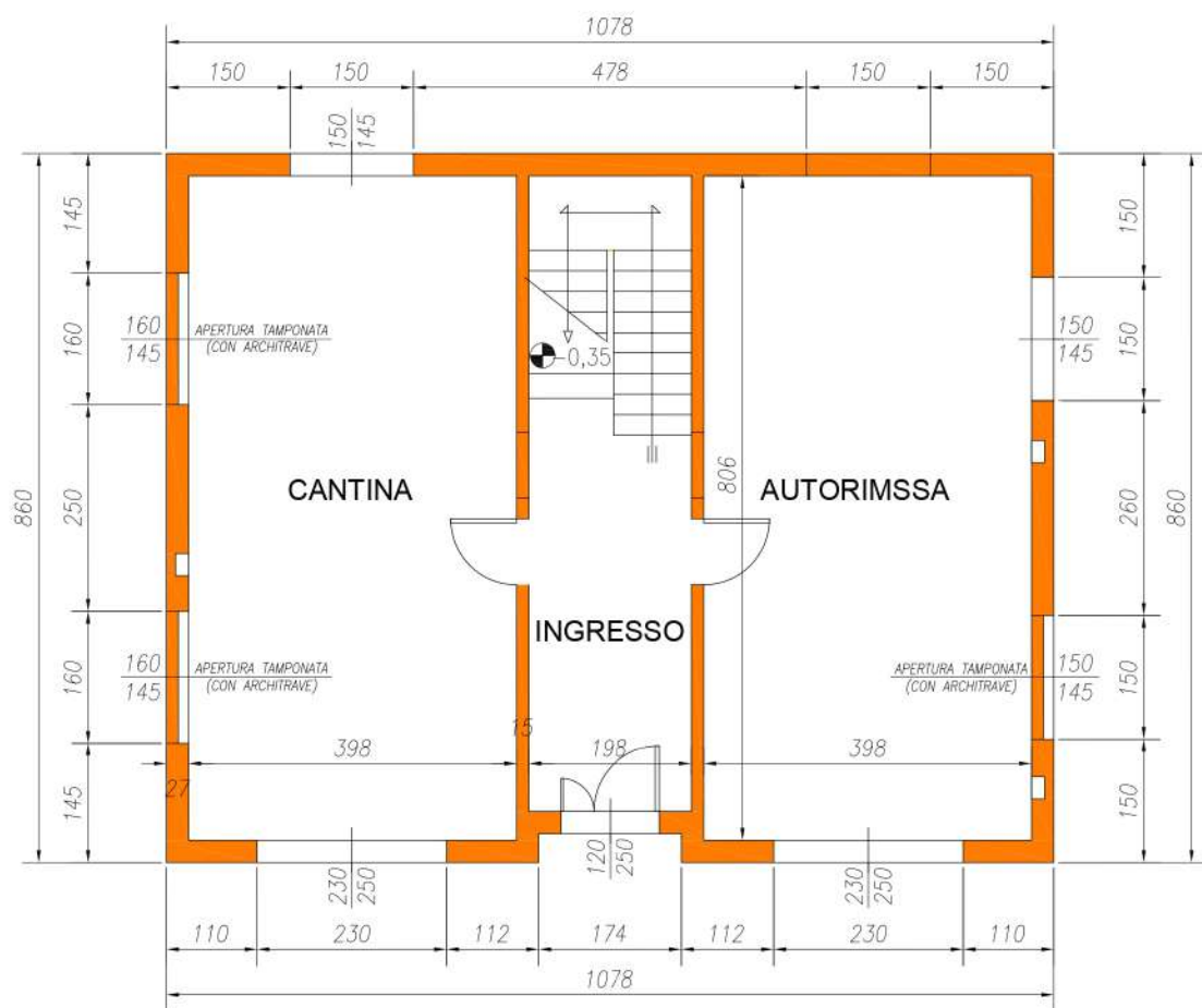
PIANO TERRA (STATO ATTUALE)
