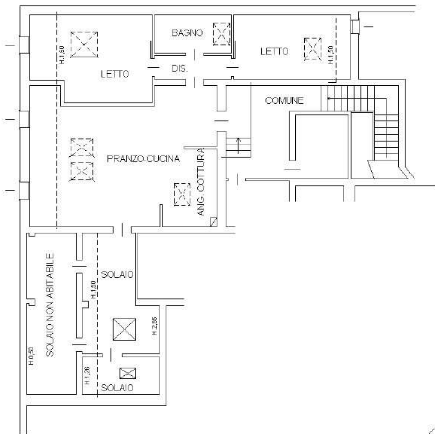
PIANTA PIANO TERZO (sottotetto) h. media 2,70
