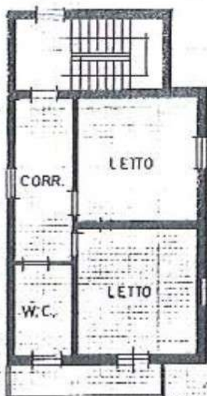
PIANO PRIMO h: 2.80
