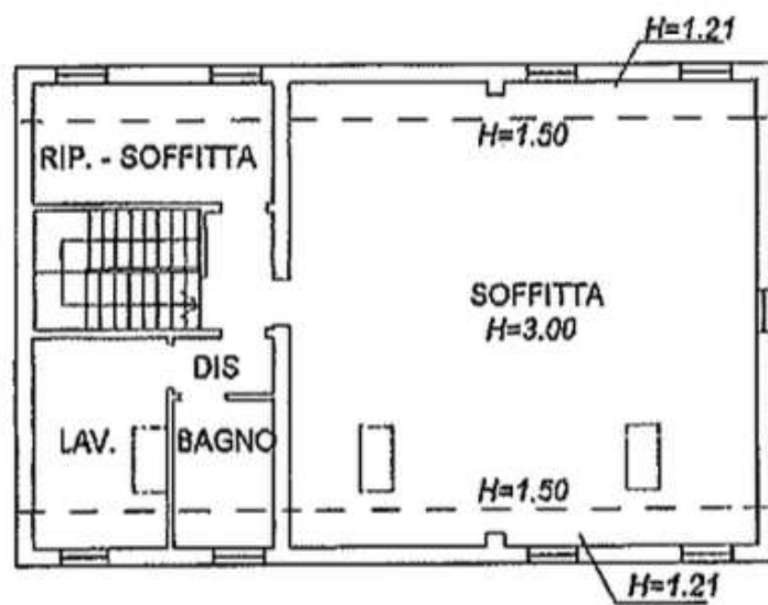
PIANTA PIANO SECONDO H.m.2.10
