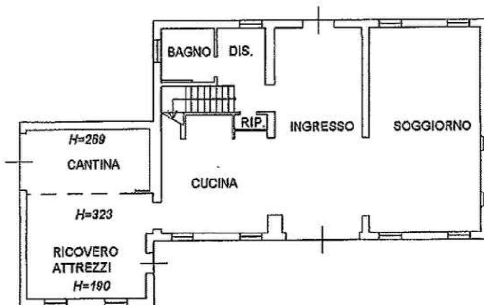
PIANTA PIANO TERRA H.2.73
