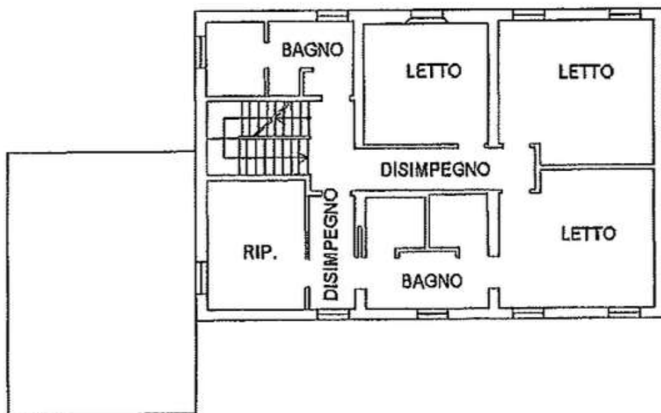
PIANTA PIANO PRIMO H.2.72
