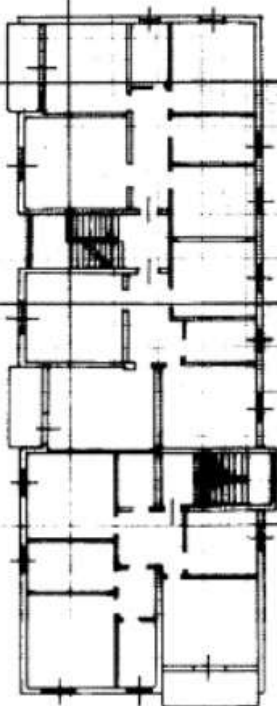
SECONDO PIANO H= 2.85
