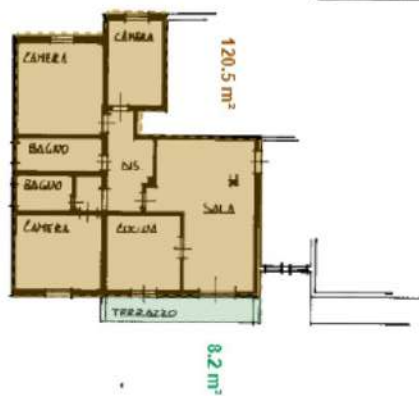
PIANO PRIMO H=2.75
