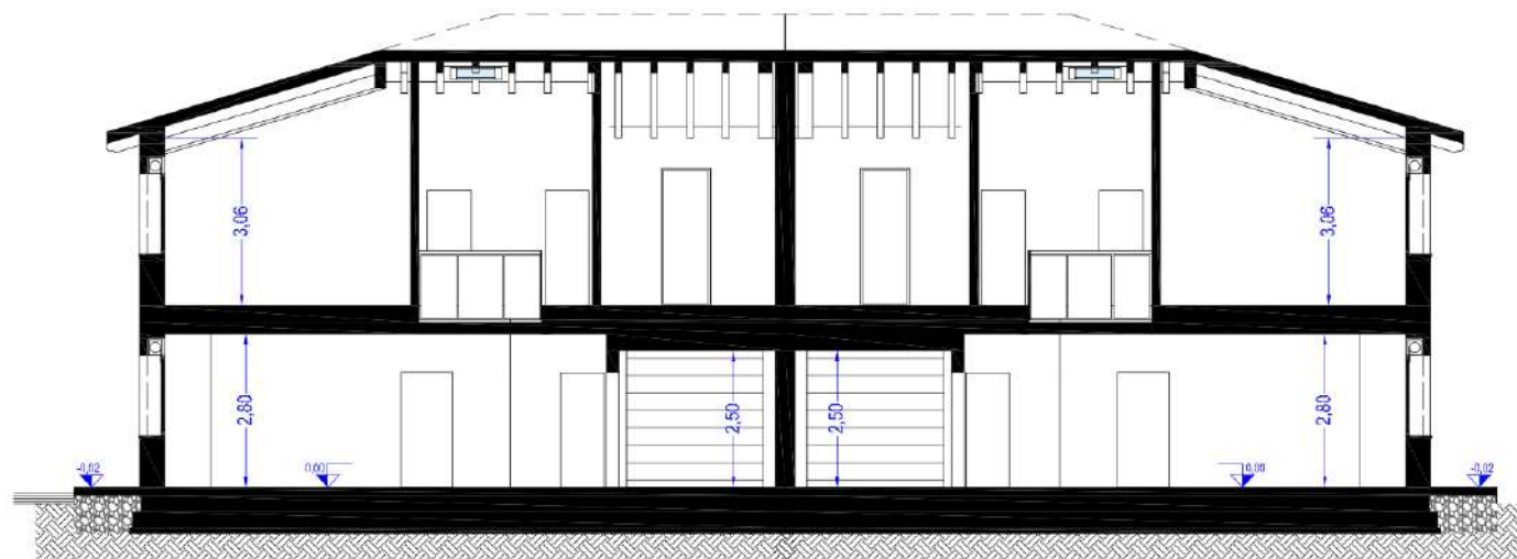
SEZIONE A
