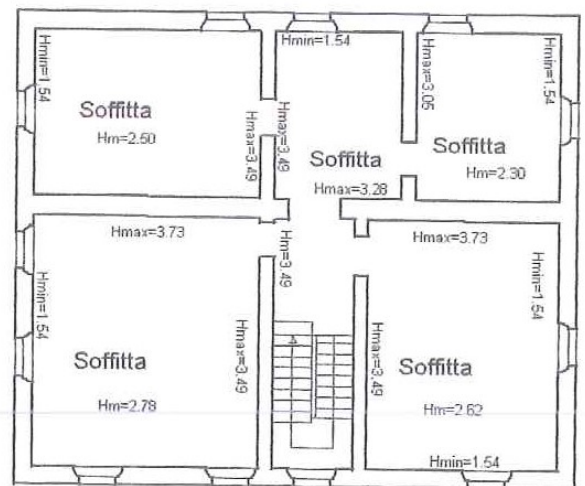
PIANTA PIANO SECONDO (Sottotetto) H=1.875
